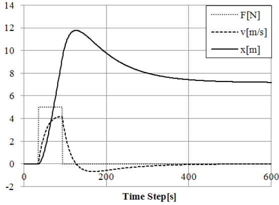
Fig. 2 Simulation of 3Element Model .
