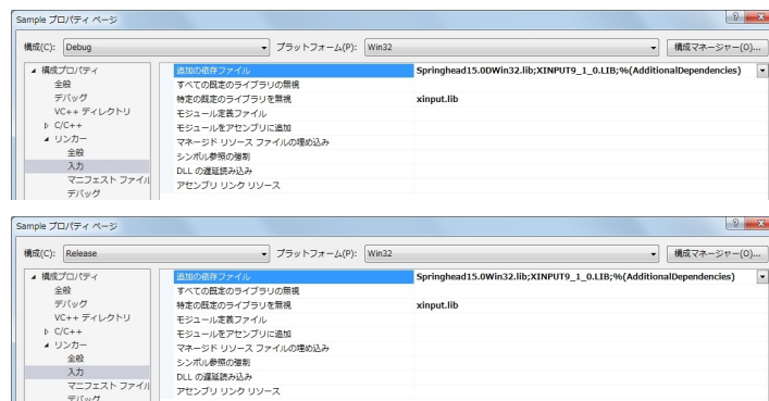
Fig. 2.7 Specify library file
