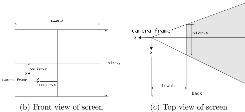
Fig. 8.3 Camera parameters
